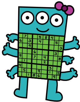
Sue Doku
